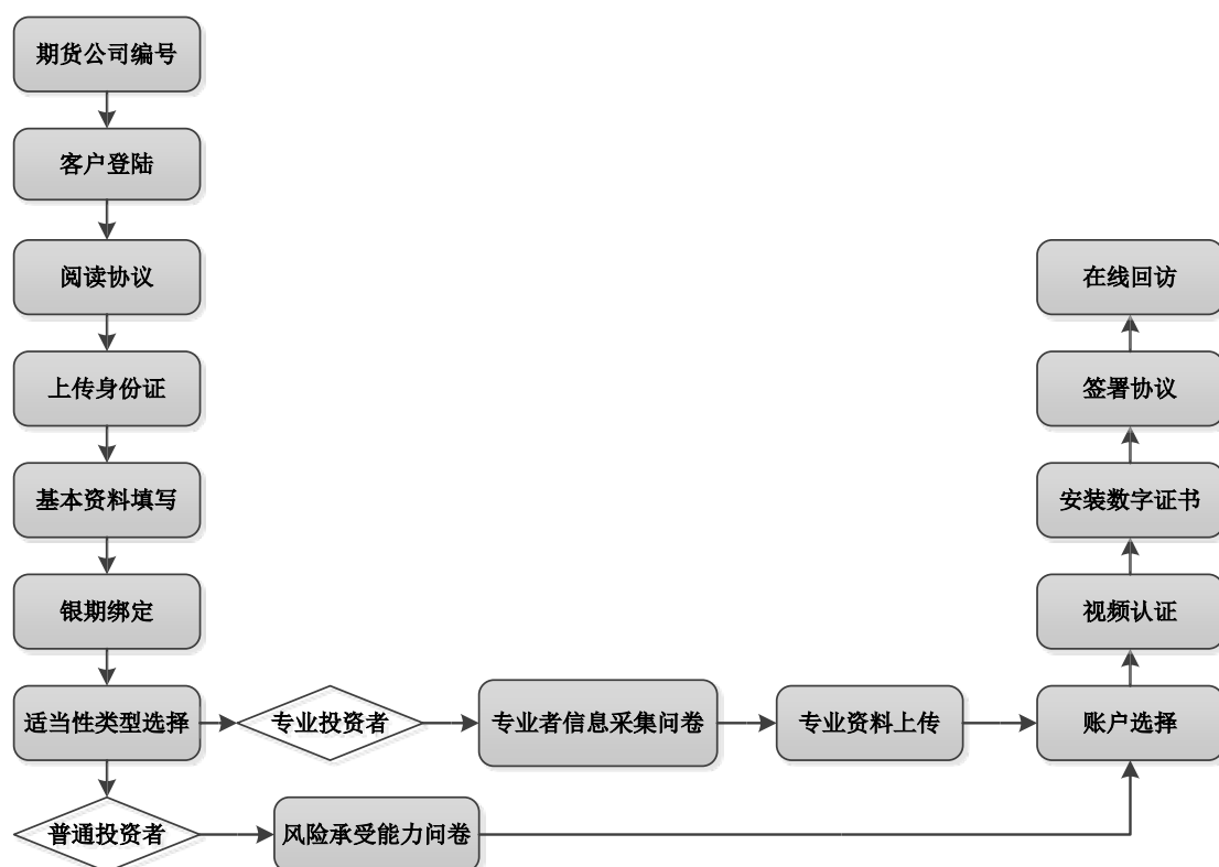
图 1 前端开户流程
