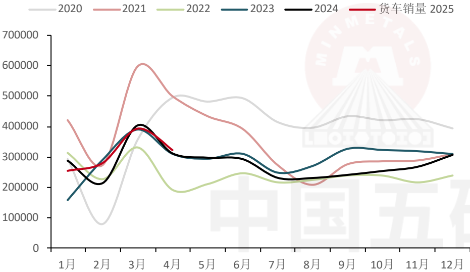
图17：货车销量(辆)
