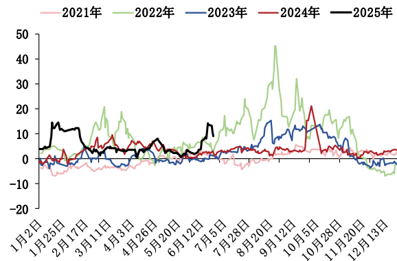
图 6：SC 原油 M1-M2 月差（元/桶）
