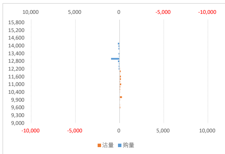
合成橡胶期权2507月份合约成交量分布
