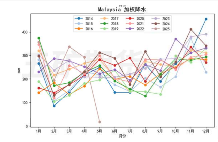
图18：马来西亚产区加权降水叠加预报至20250503（mm）
