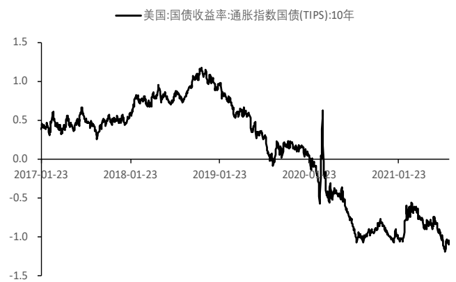
图 10：TIPS 走势
